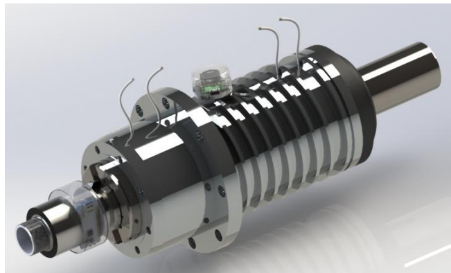
Fig 1. 工具機智慧主軸之熱特徵辨識。
